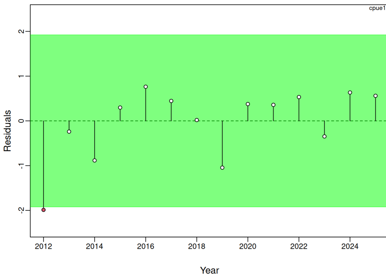
Рисунок 15 – Диагностика невязок индекса улова-на-усилие относительно теоретических оптимальных величин продукционного моделирования.
