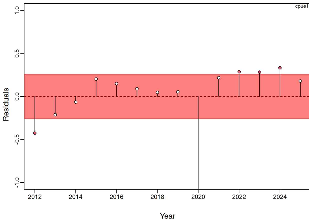
Рисунок 8 – Диагностика невязок индекса улова-на-усилие относительно теоретических оптимальных величин продукционного моделирования.
