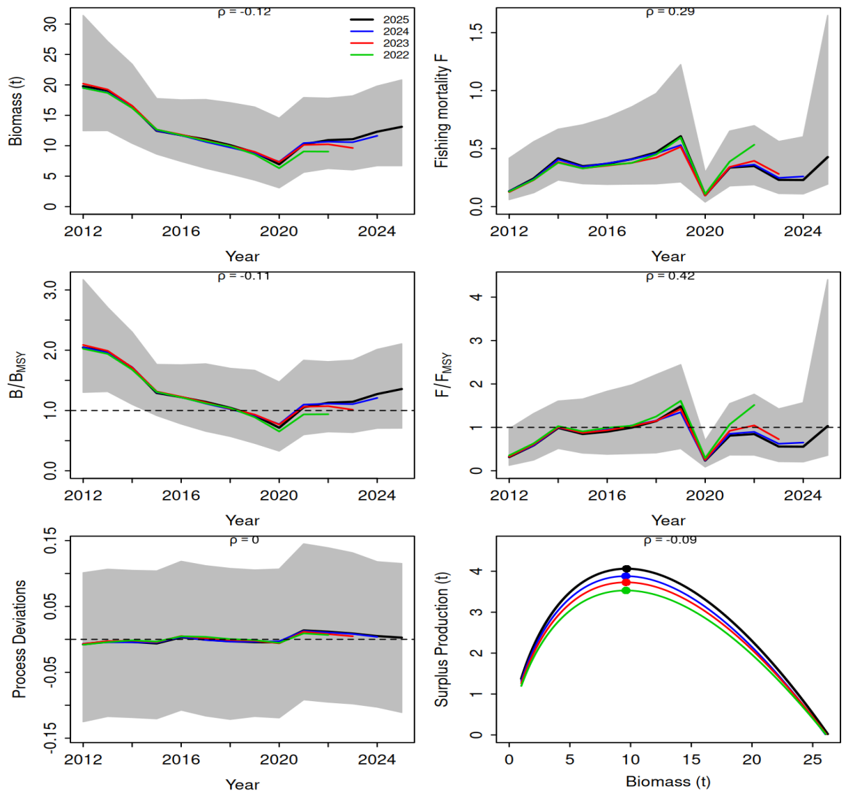
Рисунок 7 – Ретроспективный тест надежности модели с горизонтом 3 года.
