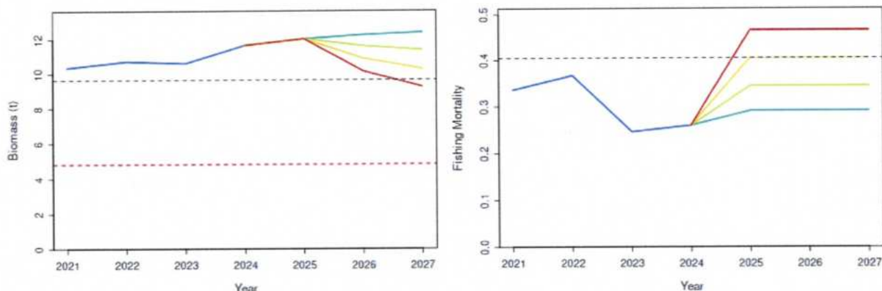
Рисунок 6 – Прогнозные сценарии состояния биомассы запаса (слева) и промысловой смертности (справа) относительно целевых ориентиры (и граничного ориентира B_{lim} – красная пунктирная линия). Синяя кривая – ретроспективные оценки, бирюзовый цвет - сценарий SQ (статус кво), желтый цвет – сценарий MSY, салатовый цвет кривой - MSY -15 %, красный цвет кривой - сценарий MSY +15 %.
