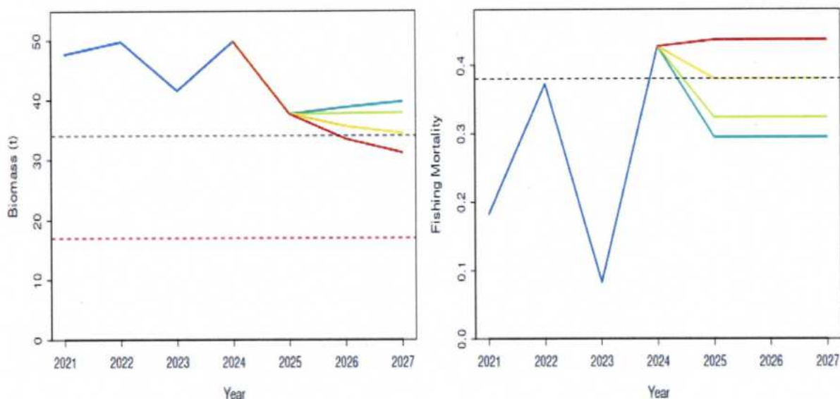
Рисунок 13 – Прогнозные сценарии состояния биомассы запаса (слева) и промысловой смертности (справа) относительно целевых ориентира (и граничного ориентира B_{lim} – красная пунктирная линия). Синяя кривая – ретроспективные оценки, бирюзовый цвет – сценарий SQ (статус кво), желтый цвет – сценарий MSY, салатовый цвет кривой – MSY -15%, красный цвет кривой - сценарий MSY +15 %.
